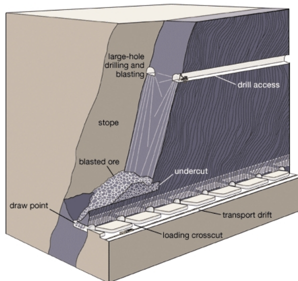
Sublevel longhole stopping
